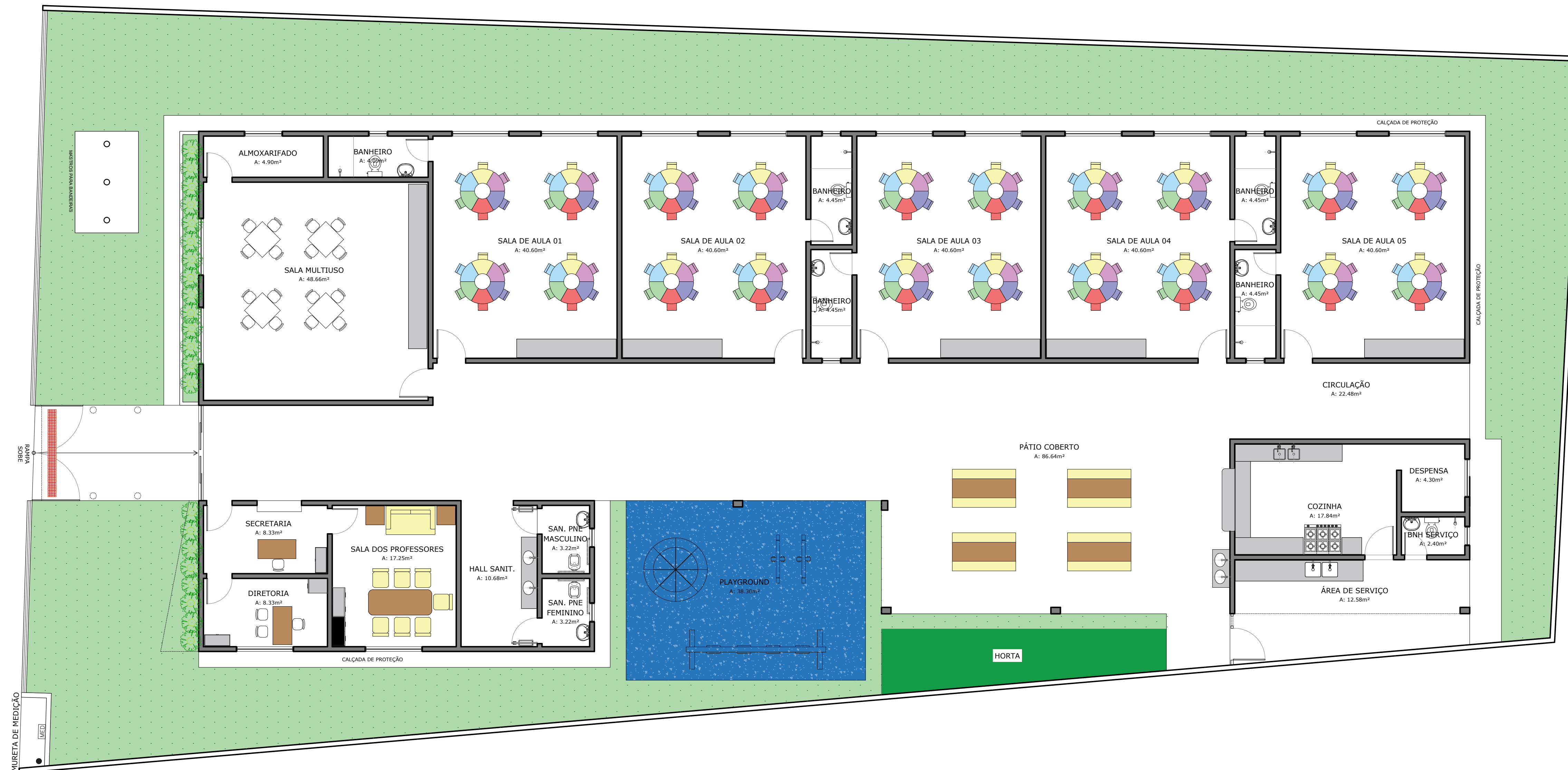
LAYOUT - CRECHE CRIANÇA ESPERANÇA ESC.: 1/75
